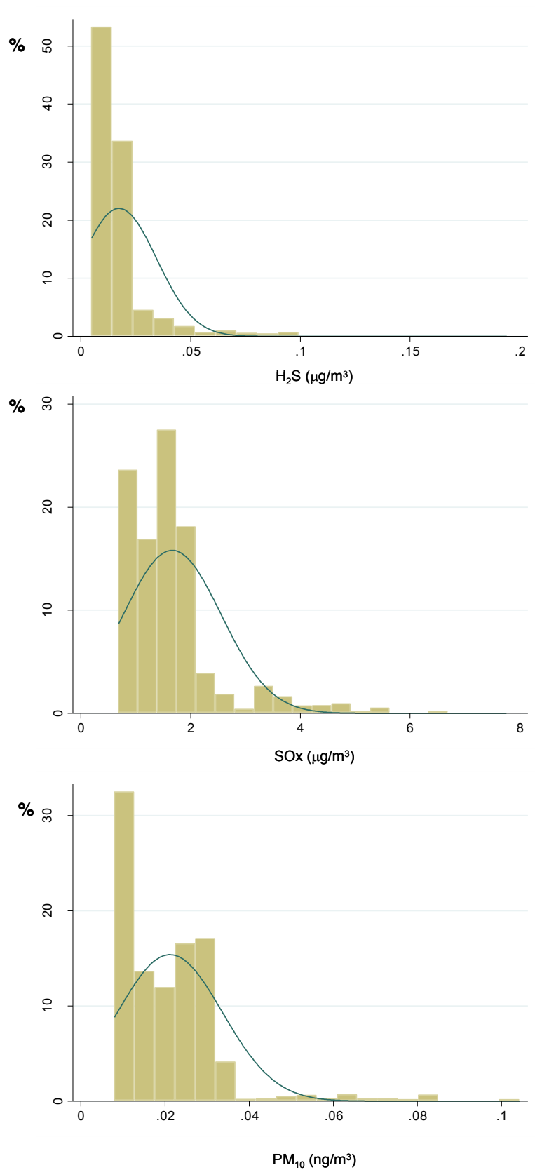
Figura 2. Distribuzione della popolazione per concentrazione di inquinante: \text{H}_2\text{S} ( \mu\text{g}/\text{m}^3 ) dalla discarica, \text{SO}_x ( \mu\text{g}/\text{m}^3 ) dalla raffineria e \text{PM}_{10} ( \text{ng}/\text{m}^3 ) dall'inceneritore per rifiuti speciali
